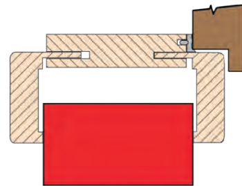
ŠTANDARDNÁ OBLOŽKOVÁ ZÁRUBŇA
