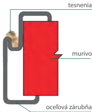
PROFIL OCEĽOVEJ ZÁRUBNE PRE DPB 3
